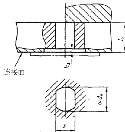
图 6 扁头驱动件示意图
