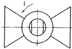
图 11 被驱动件扁头的位置
