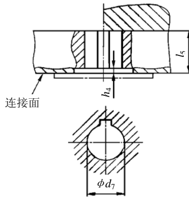
图 3 键连接驱动件示意图
