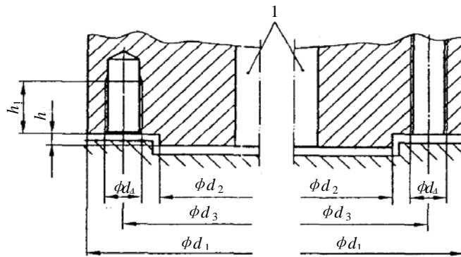
图1 驱动装置与阀门的连接示意图
