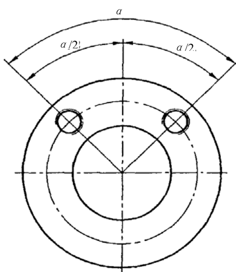
图2 螺纹（孔）位置
