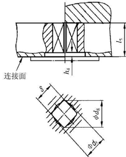
图 5 对角方头驱动件示意图
