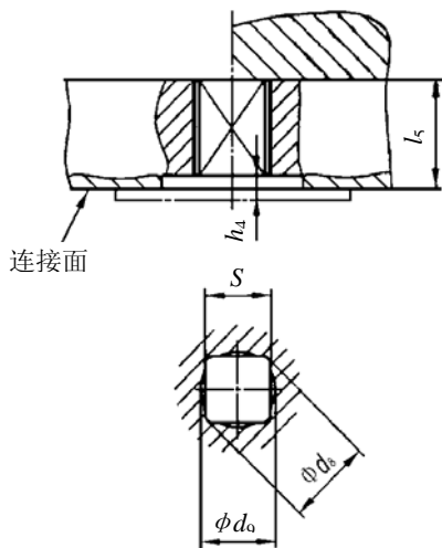
图 4 平行方头驱动件示意图
