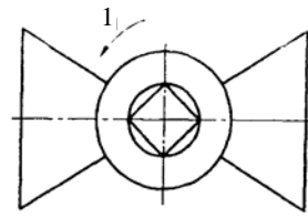
图 10 被驱动件对角方头的位置
